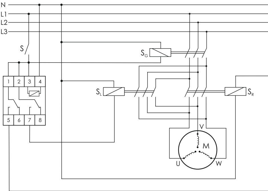
S G – основной контактор; S R , S L – контакторы переключения обмоток.
